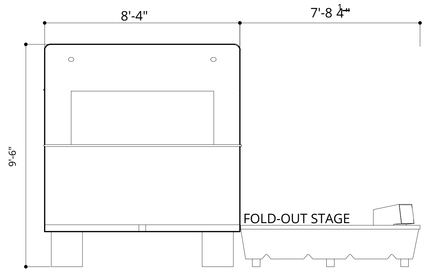
The Etta Front Elevation
