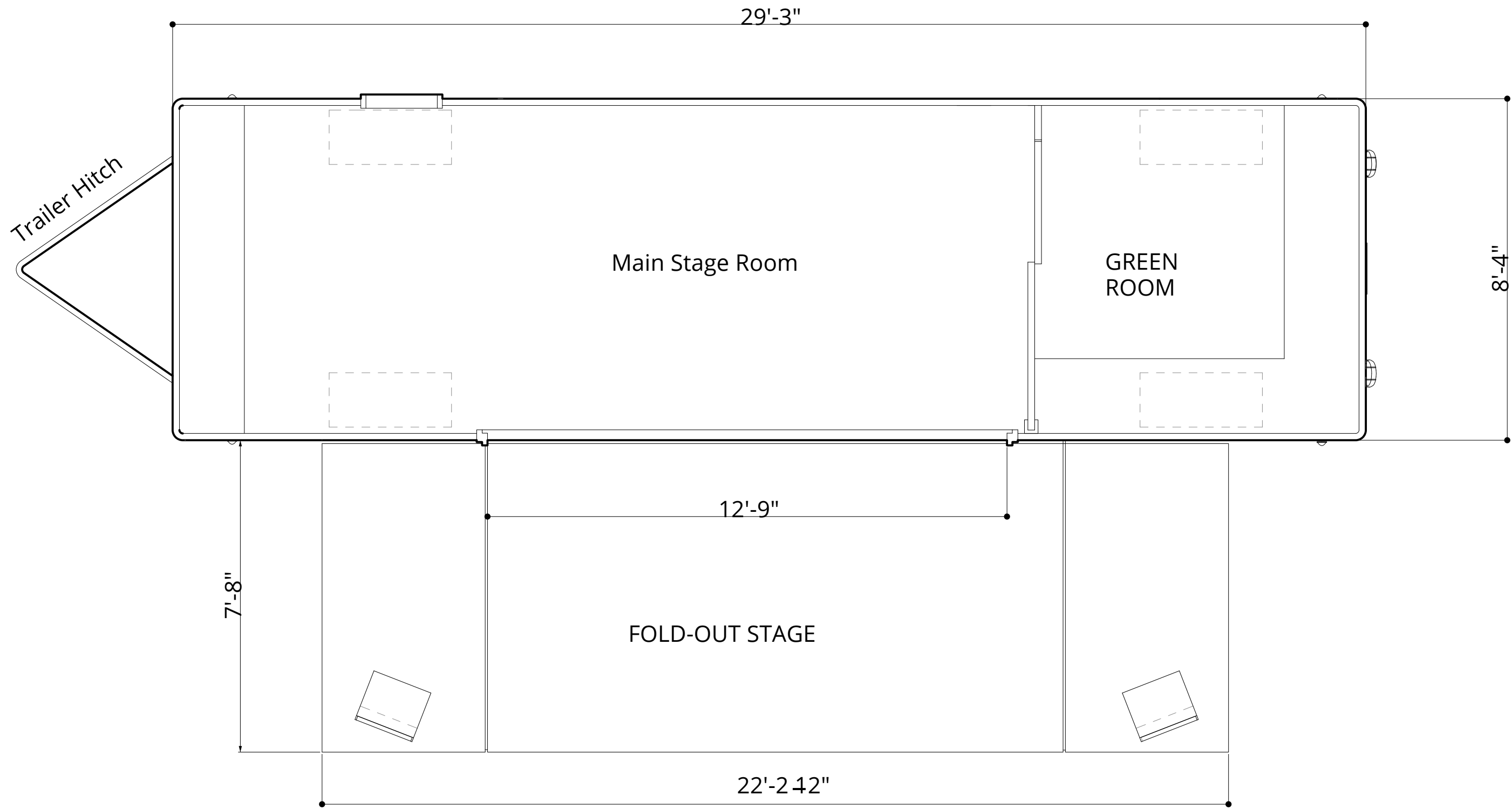
The Etta Plan
