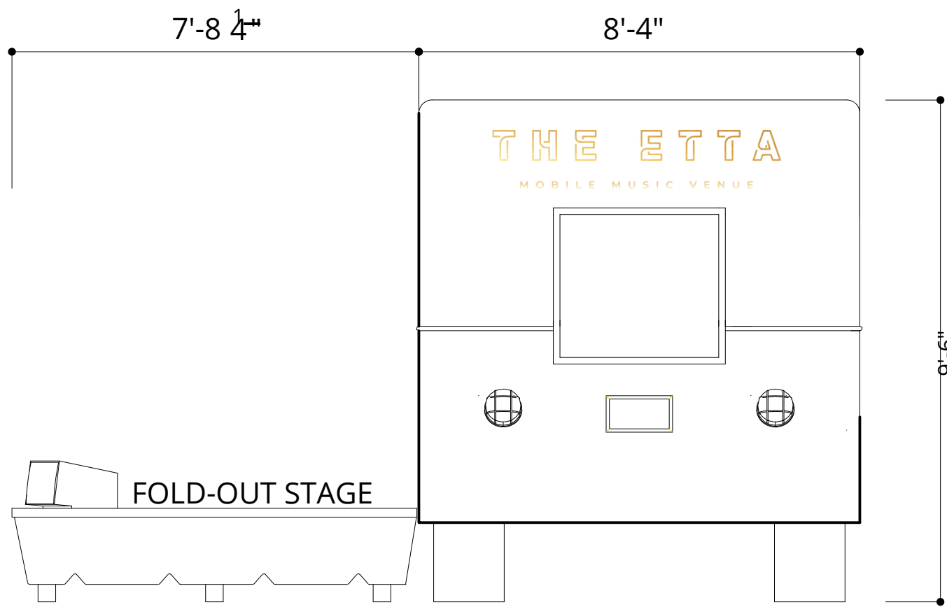
The Etta Back Elevation
